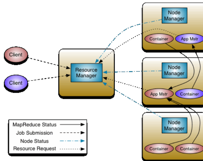
Figura 6: Arquitectura de YARN en Hadoop
